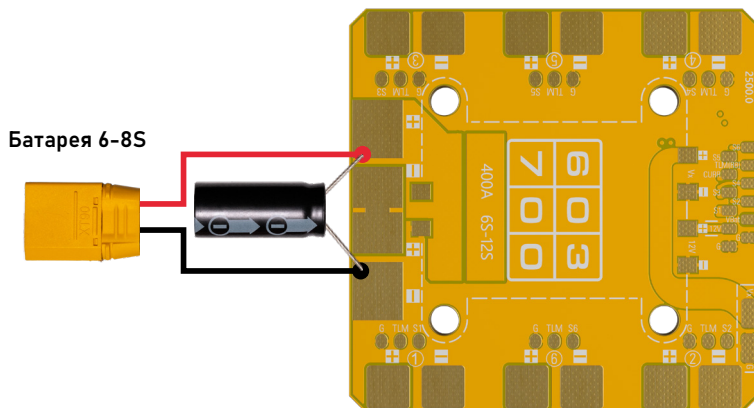
Схема підключення живлення 6-8S
