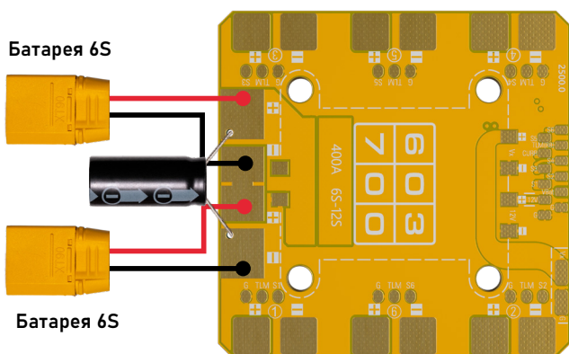
Схема підключення живлення 12S
