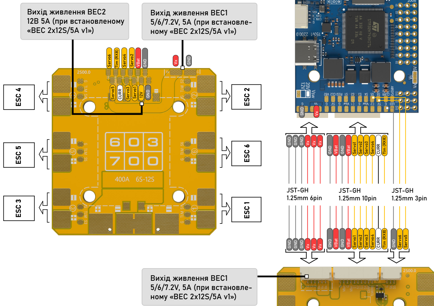
Схема підключення живлення 6-8S
